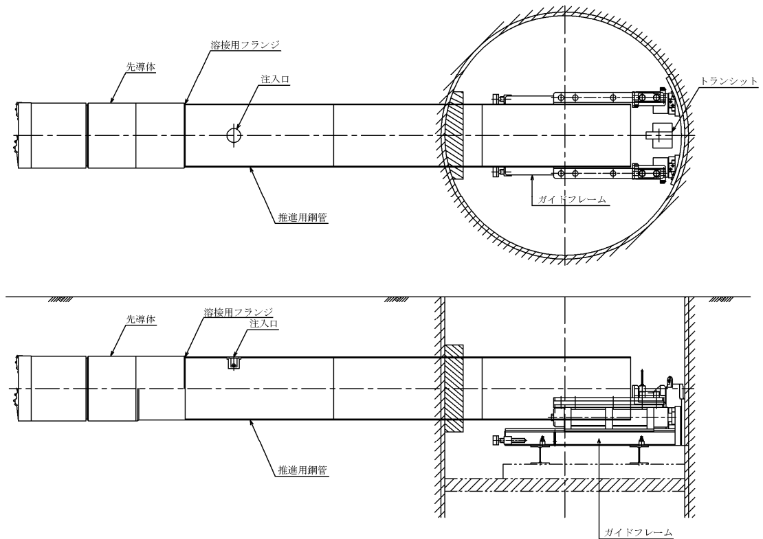
(2) 平面・縦断面図
