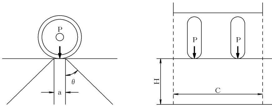
図 6-6-2 後輪荷重の分布
