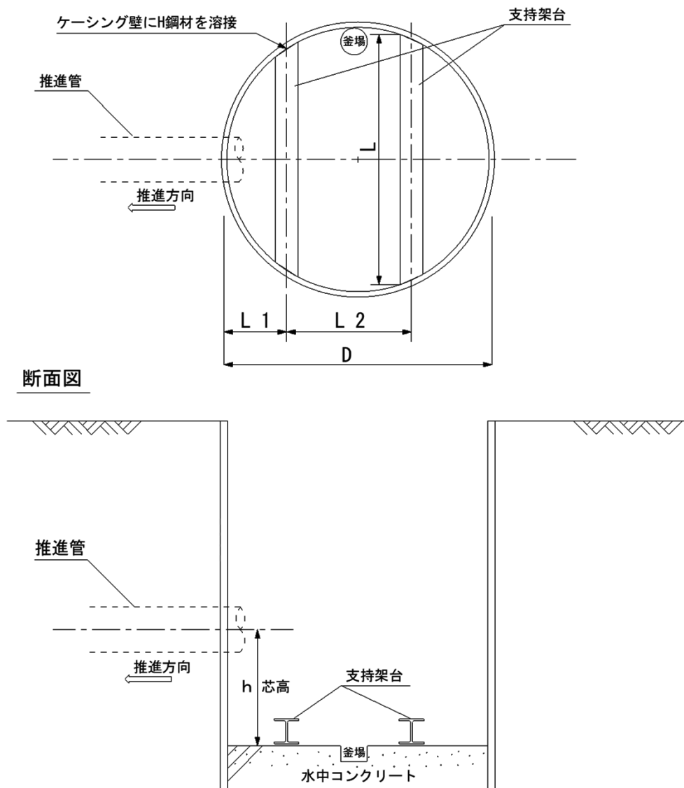
図-15 小型立坑（鋼製ケーシング方式）
