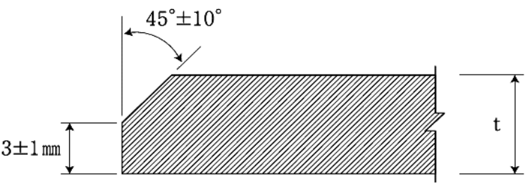
図-8 ベベル加工図
