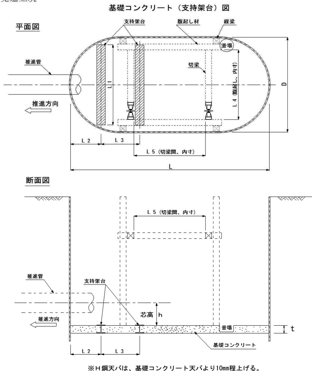
図－13 小判形発進立坑
